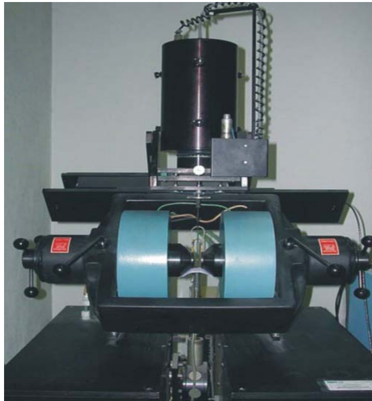
Figure 18 : Exemple de magnétomètre à échantillon vibrant VSM permettant de mesurer l'aimantation en fonction du champ appliqué sur une large gamme de champ ( \pm 1\text{T} ). Source http://auracenter.fr/Art/D%C3%A9tection.html
